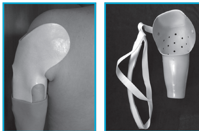
Slika 4: Definitivno z menjajočimi se področji pritiskov in razbremenitev (a) in ležišče z ramensko kapo (b).
