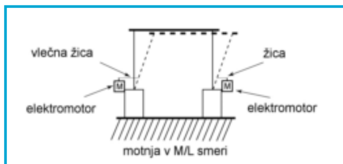
Slika 2: Naprava povzroči nenadno mehansko motnjo v medialno-lateralni (M/L) smeri v višini bokov. Oseba v napravi se na motnjo odzove s posturalnim odzivom, ki preprečuje padec.
